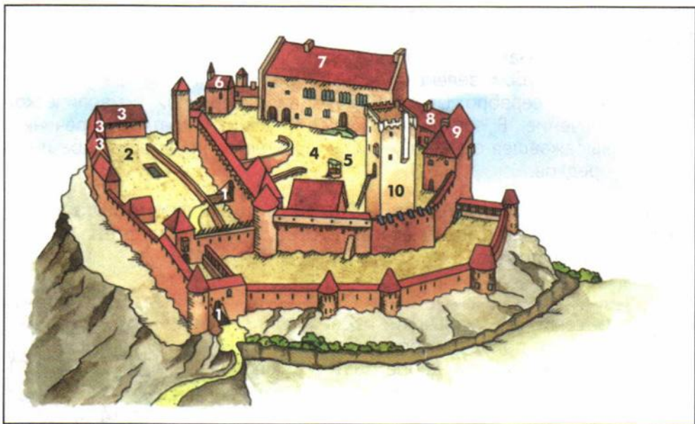
План рыцарского замка. Современная реконструкция: 1 — подъёмный мост; 2 — нижний двор; 3 — конюшня, хлев, амбары; 4 — верхний двор; 5 — колодец или резервуар с водой; 6 — замковая часовня; 7 — жилище хозяина; 8 — помещение для хранения оружия и доспехов; 9 — жилые помещения; 10 — донжон
