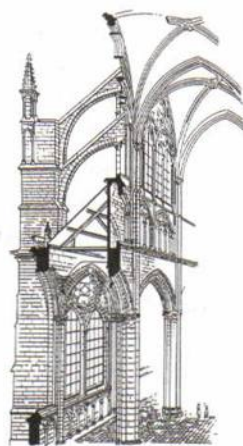
Схема готического храма в разрезе
